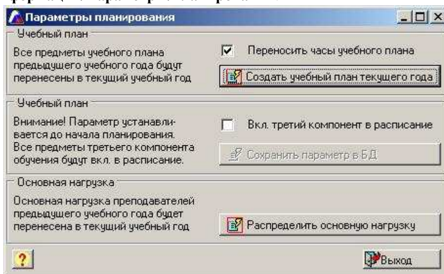
Рис. Окно «Параметры планирования»
