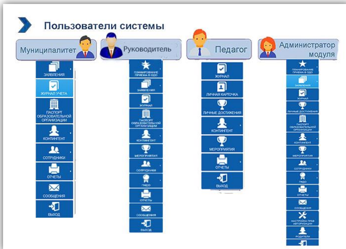
Рис 1.1 Пользователи системы
