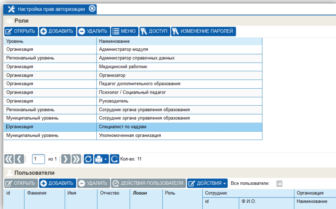
Рис 1.2. Пользователи системы
